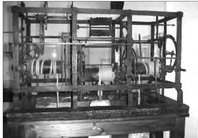
Weidaer Rathausuhrwerk von Melchior Steinmüller 1669
