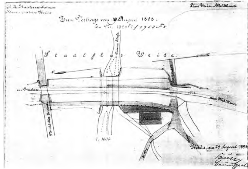
Lageplan zum Bau des Elektrizitätswerkes Weida an der Schloßmühle
